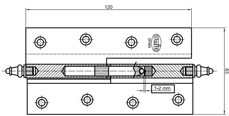
Mod. 1207-120 IZQUIERDA
