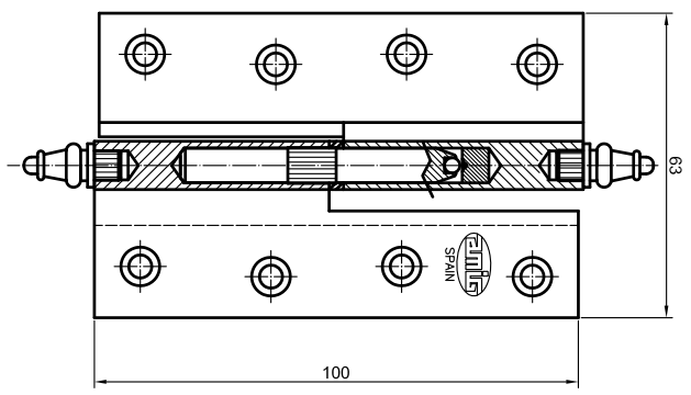
Mod. 1207-100 DERECHA
