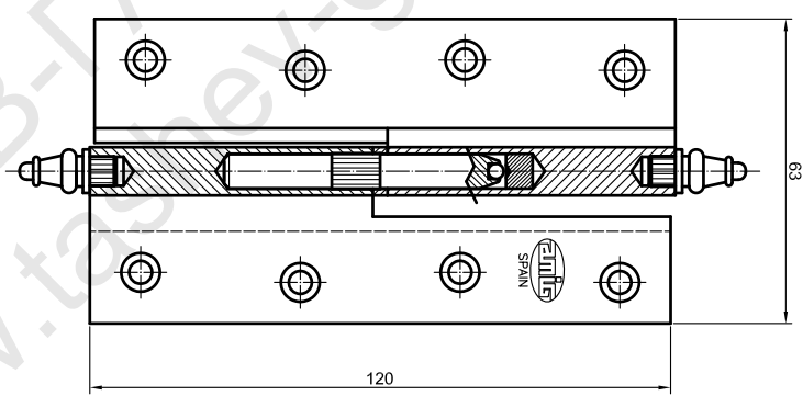
Mod. 1207-120 DERECHA
