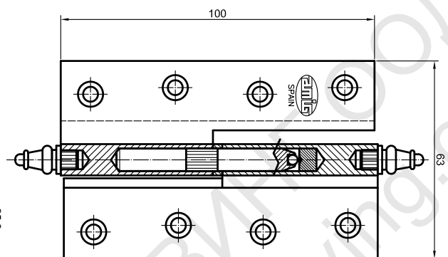
Mod. 1207-100 IZQUIERDA
